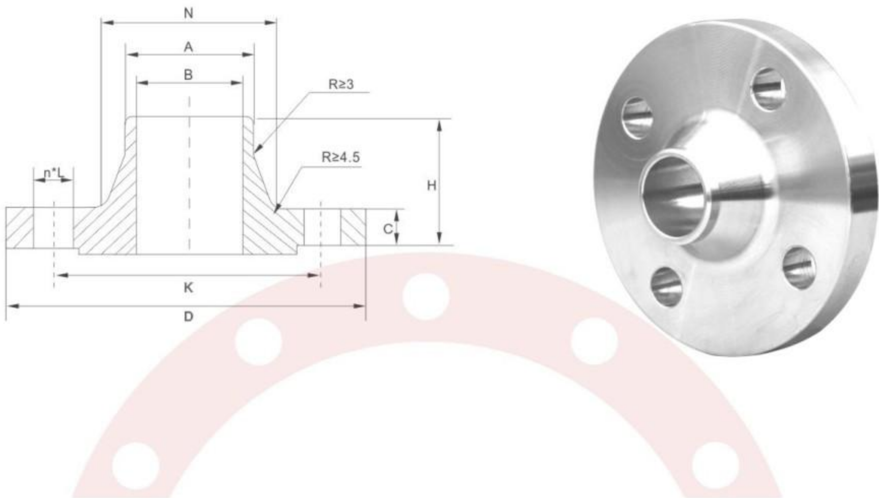
Class150(PN20) 带颈对焊钢制管法兰 (mm)
