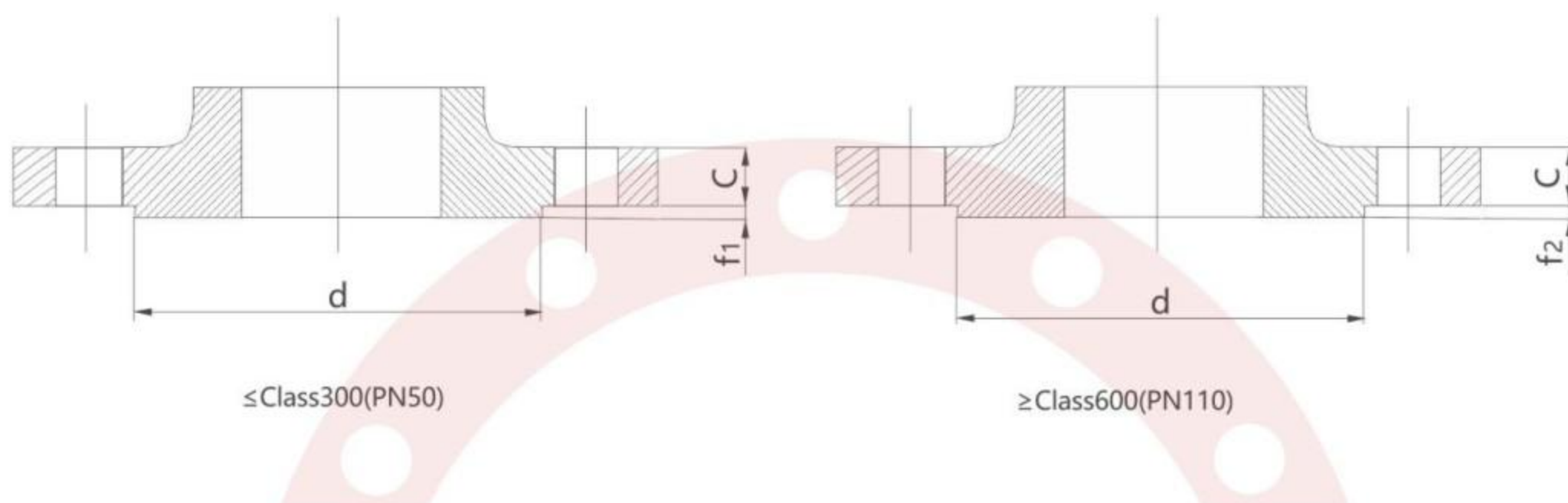
突面法兰 (RF) 面的密封面尺寸
