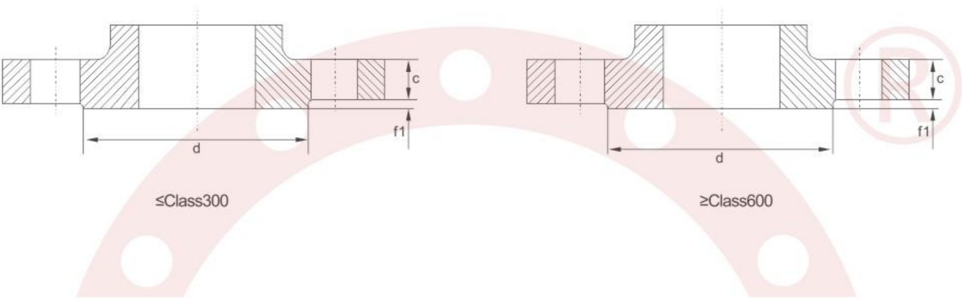
A系列大直径法兰的密封面尺寸突面 (RF) (mm)
