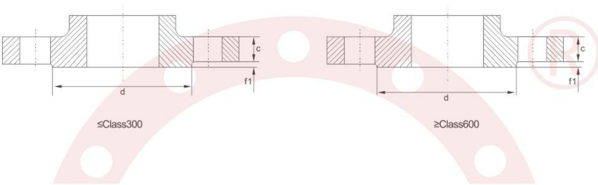
B系列大直径法兰的密封面尺寸突面 (RF) (mm)
