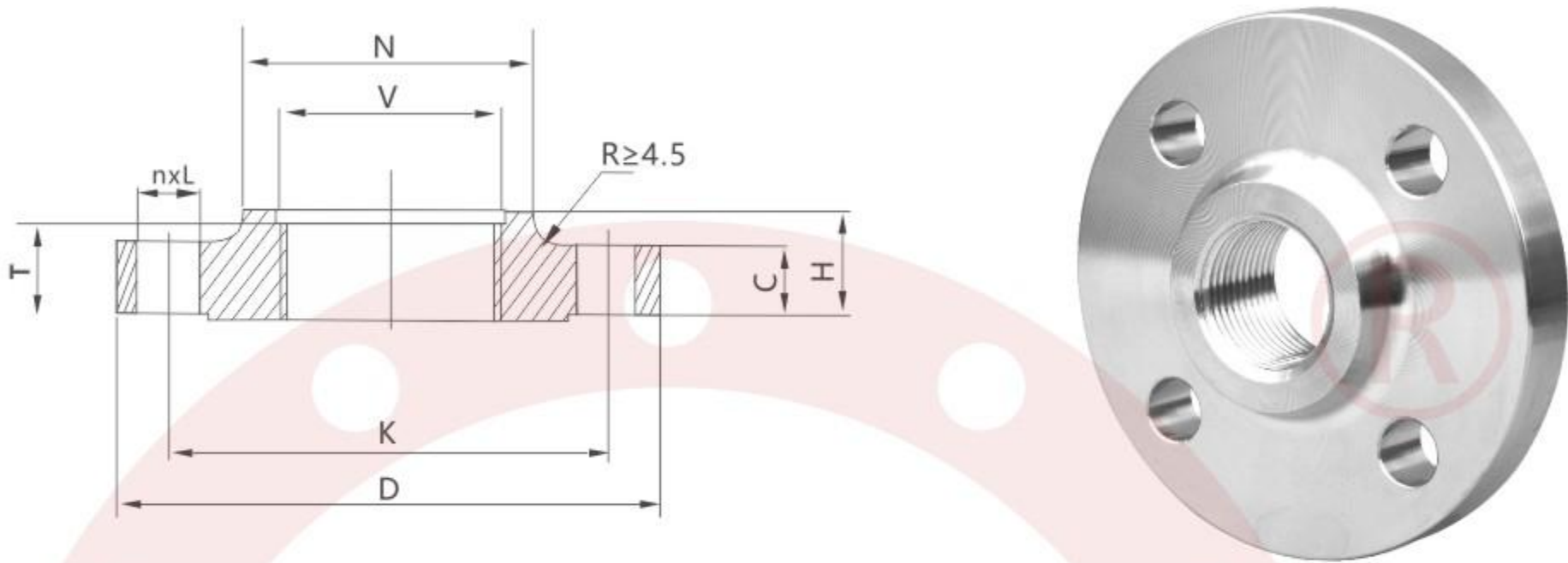
Class150(PN20) 螺纹钢制管法兰
